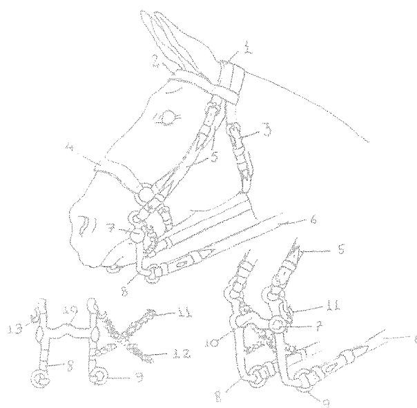
Fig 03 Cabeçada de freio
